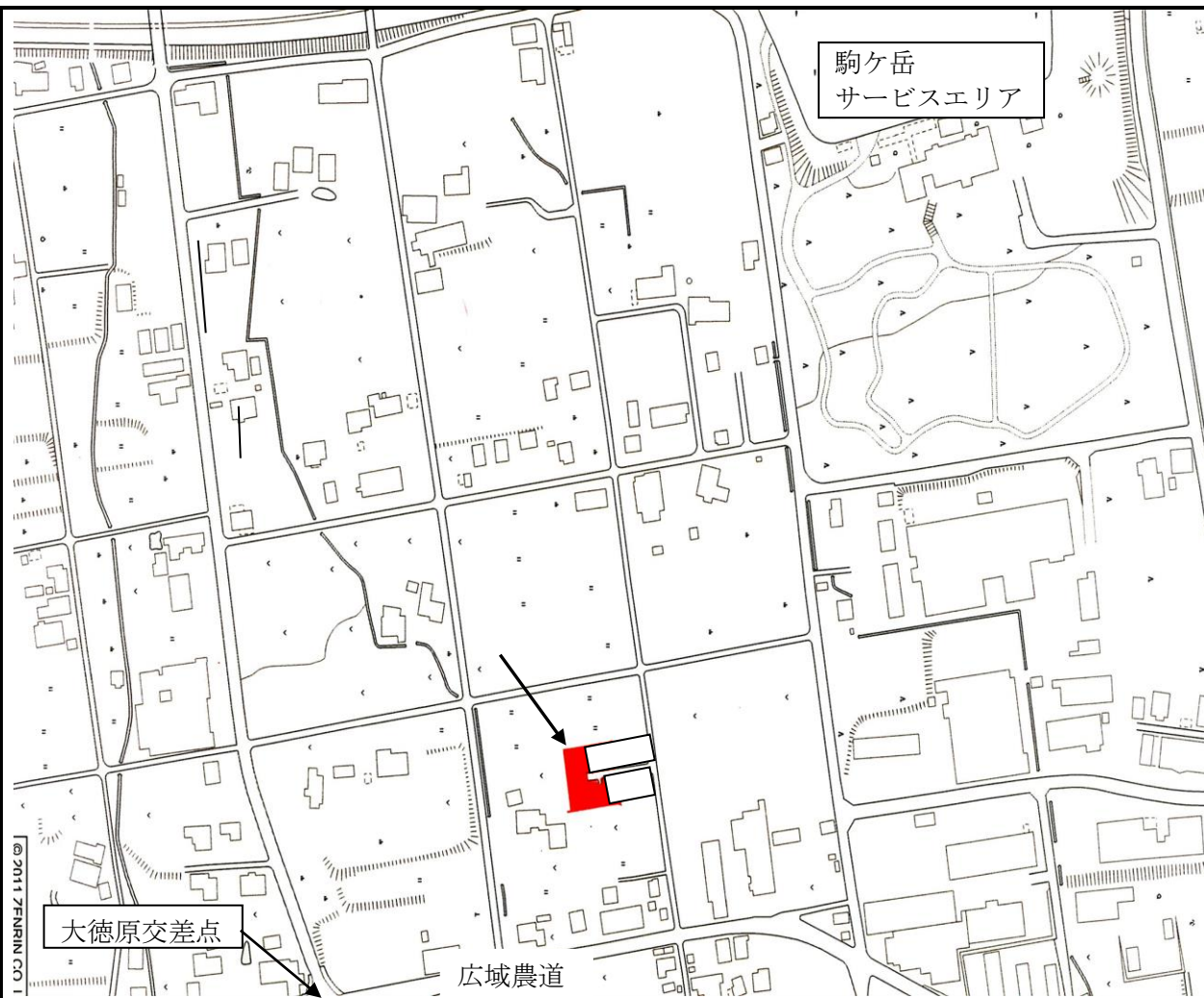
【 案内図 】
